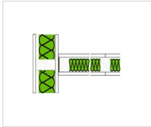
T-ANSCHLUSS
