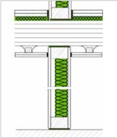
ANSCHLUSS AN MASSIVHOLZDECKE
