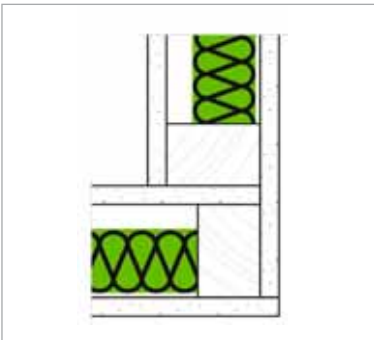
ECKAUSBILDUNG
