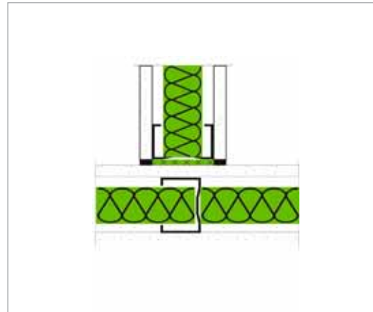
T-ANSCHLUSS
