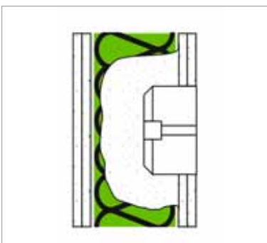
BRANDSCHUTZTECHNISCHER EINBAU STECKDOSE MIT GIPSMÖRTEL
