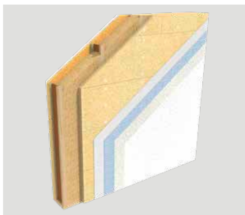
Fissaggio ai montanti diretto
