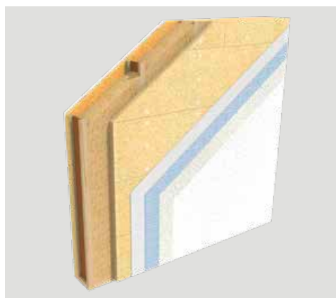
Fissaggio ai montanti indiretto
