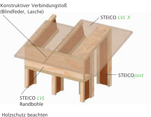
D11 Ortgang mit STEICO Furnierschichtholzplatte
