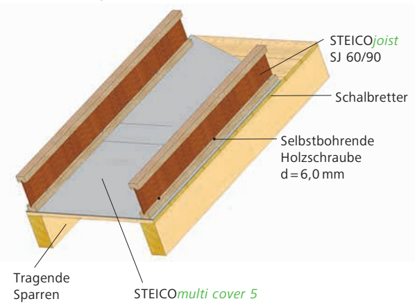
D12 Aufdachdämmung – Aufdoppelung mit STEICOjoist
