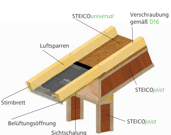
D8 Traufe mit Luftsparren nicht sichtbar
