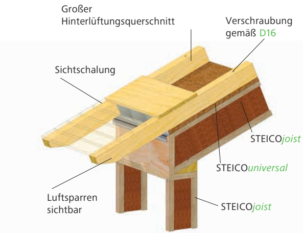
D7 Traufe mit Luftsparren sichtbar
