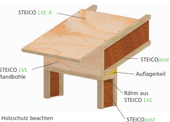
D11 Ortgang mit STEICO Furnierschichtholzplatte
